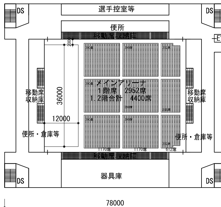
1階床面積 4768㎡ (1~2階床面積合計 7128㎡) メインアリーナ 1階ブロックプランイメージ 1/800
