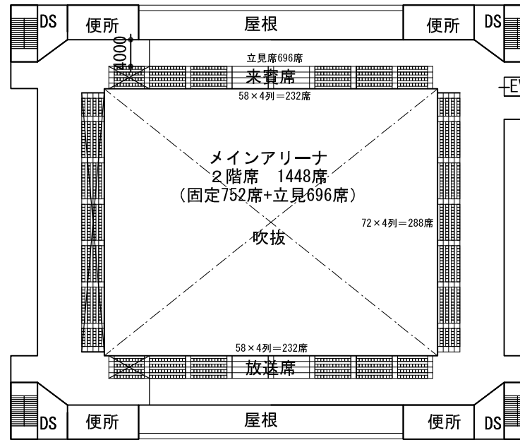
2階床面積 2360㎡ メインアリーナ 2階ブロックプランイメージ 1/800
