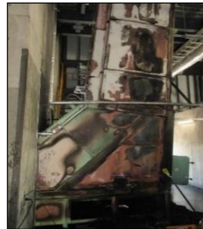
③破碎物コンベヤ（選別室1階側）
