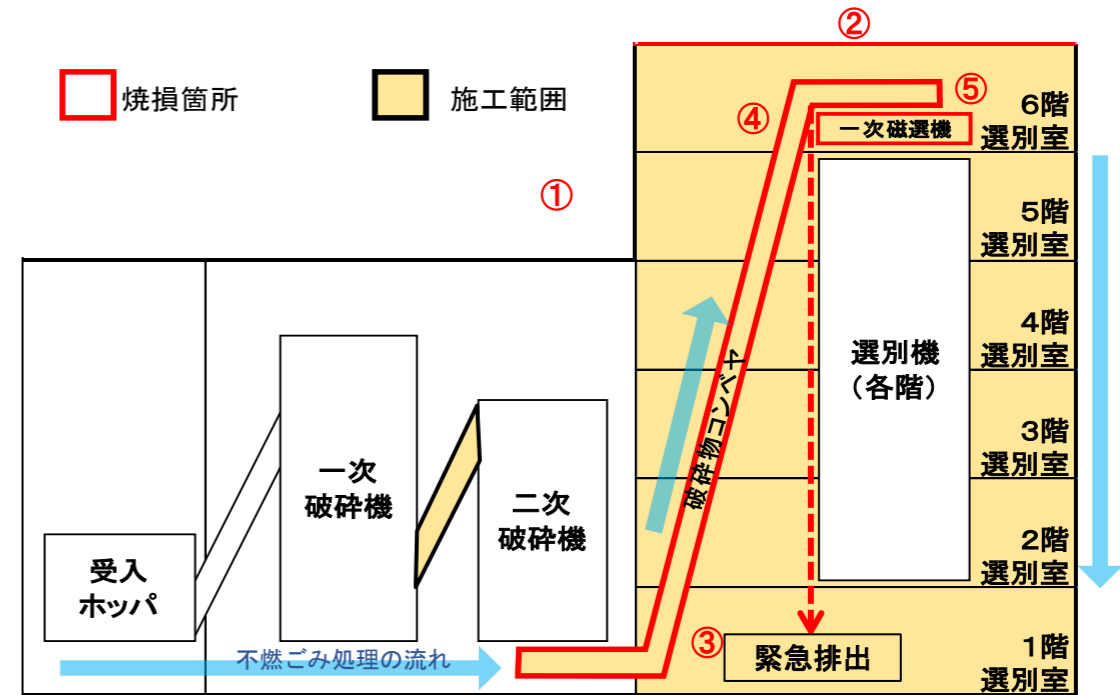
破碎選別処理施設フロー図（施工範囲）
