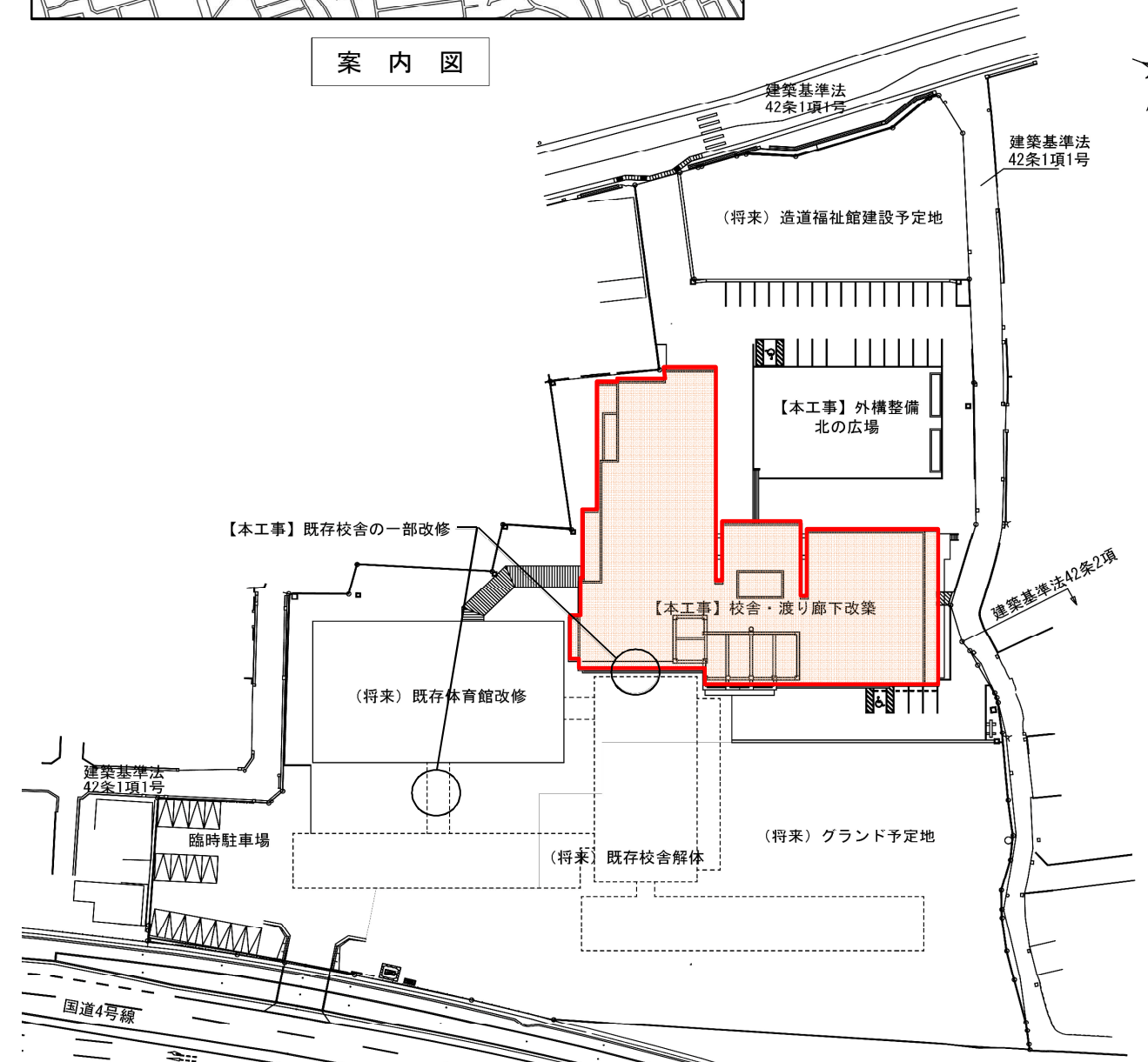
配置図
